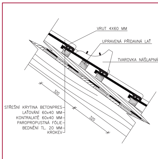
Řez usazením tvarovky nášlapné
